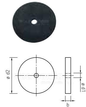
guarnizione Dichtscheibe
